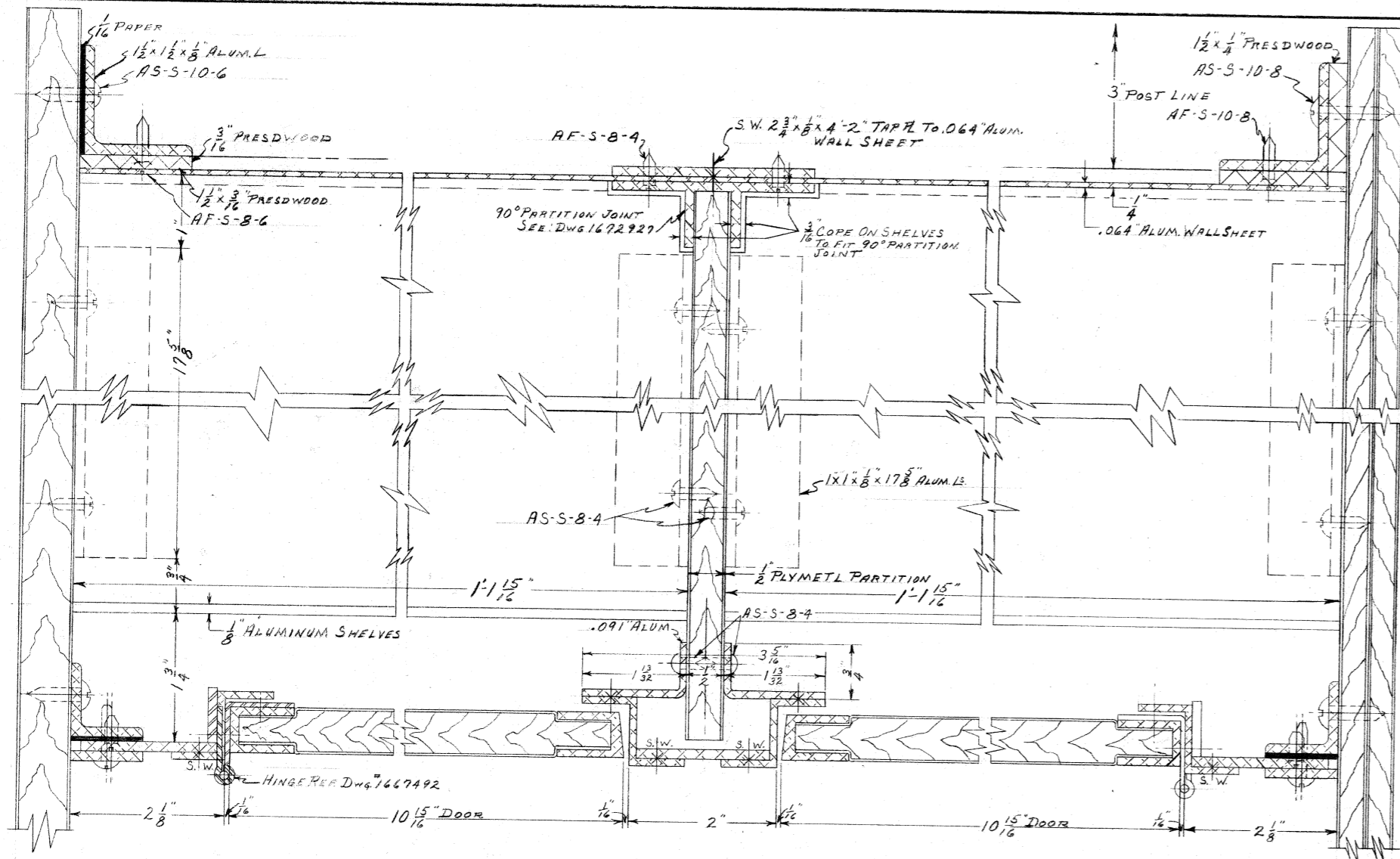
SECTION A-A
