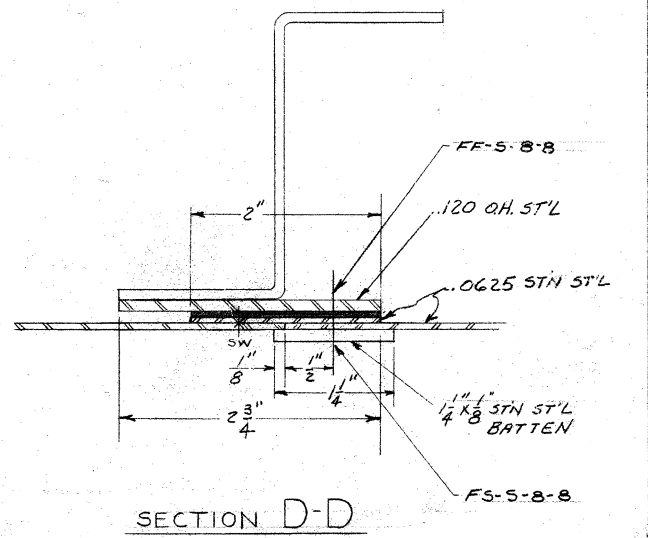
SECTION D-D
